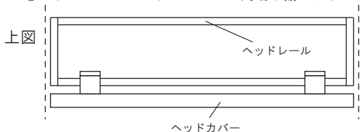
⑤ヘッドカバーとヘッドレールの両端を揃えます
