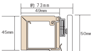
各部のサイズ
