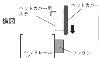
⑤ヘッドカバーとヘッドレールの両端を揃えます
