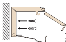
正面付けの場合
